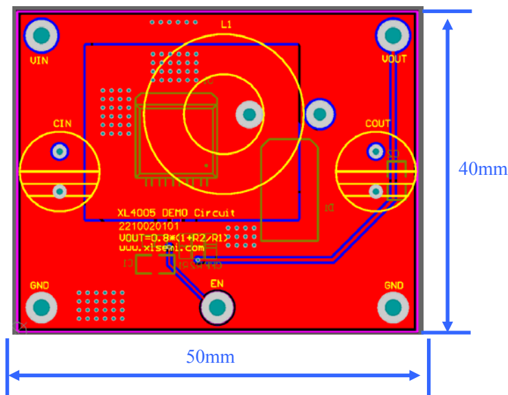
顶层
